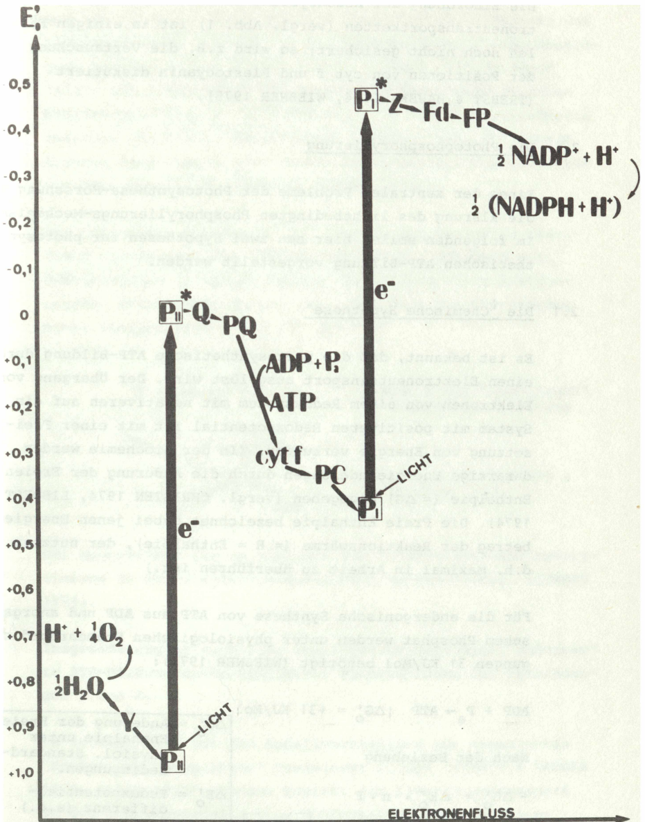
Abb. 1: Der photosynthetische Elektronentransport vom Wasser zum \text{NADP}^+ . (vergl. Tab. 1, nach WIESSNER 1975)
