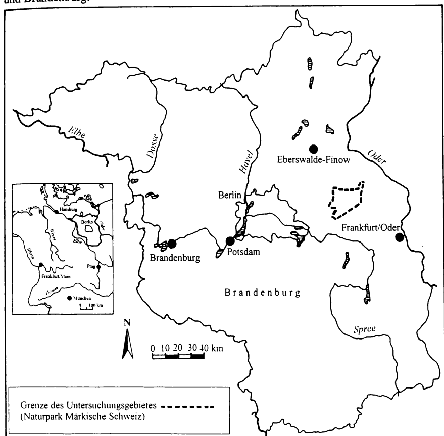
Abb. 1: Lage des Untersuchungsgebietes (Naturpark Märkische Schweiz) in Mitteleuropa und Brandenburg.
