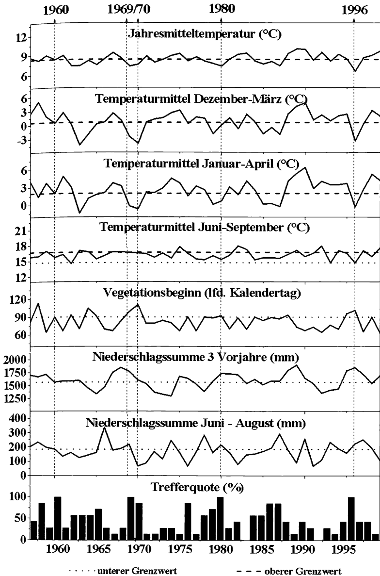
Abb. 1: Selektierte Witterungsgrößen sowie Trefferquoten bei der Einhaltung der Grenz- bzw. Optimalbereiche für das Auftreten von Zwergbinsen-Gesellschaften auf Ackerland zwischen 1957 und 1999.
