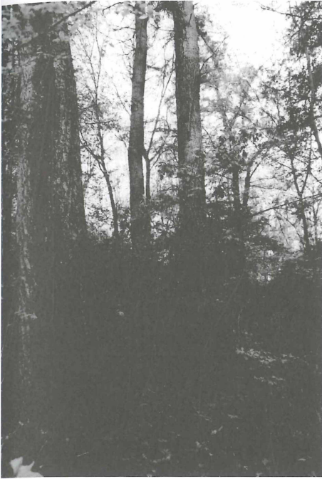
Abb. 7: Über 80-jährige Populus alba aus Wurzelbrut entstanden, Mutterbaum siehe Abb. 6, und Ulmus laevis (links). Foto: Mai 2007.
