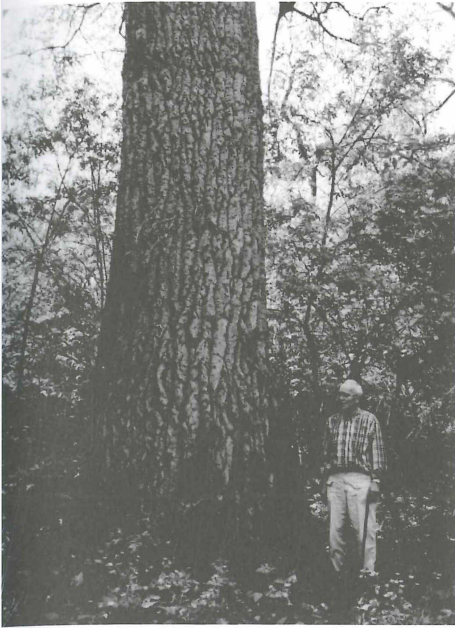
Abb. 5: Über 250-jährige Populus alba im Weichsel-Delta – ein Baum der „12 Apostel“. Foto: Mai 2007.
